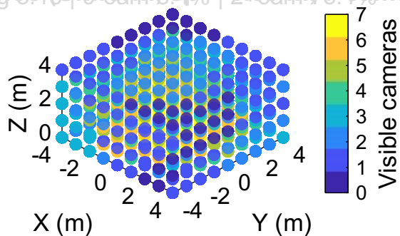
OptiTrack ad-hoc (Cost: 0.2691)
