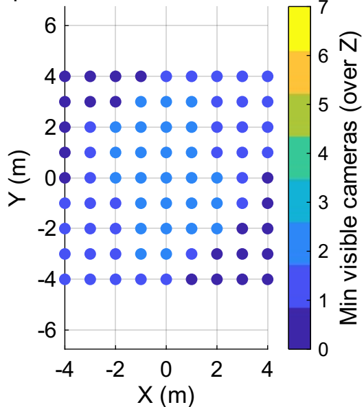
OptiTrack ad-hoc: XY worst-case
